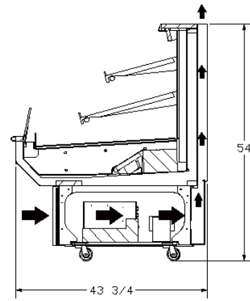
MMR-54
