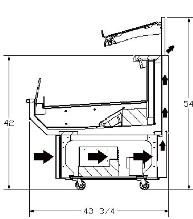
MMR-42
