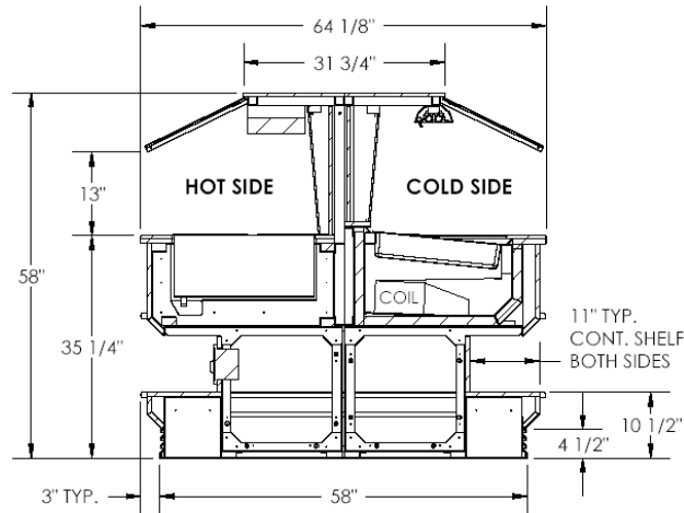
WSB-2-HC (ANGLED PANS SHOWN)
