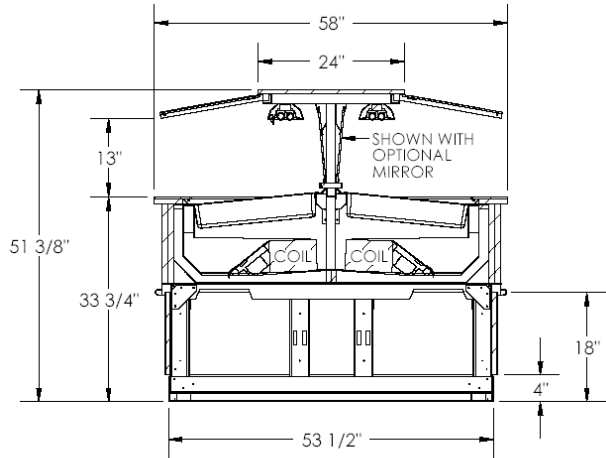
WSB-2 (ANGLED PANS SHOWN)
